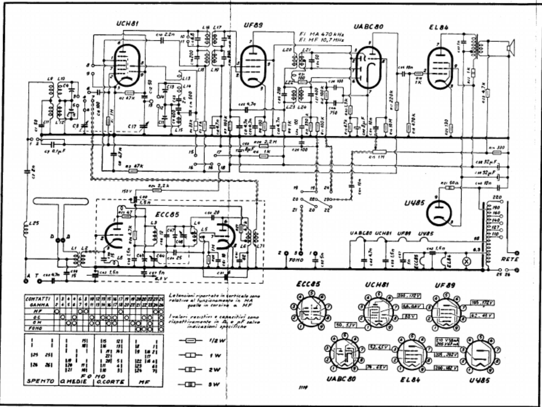
WATT RADIO - Mod. 36 MF classe Anie.
